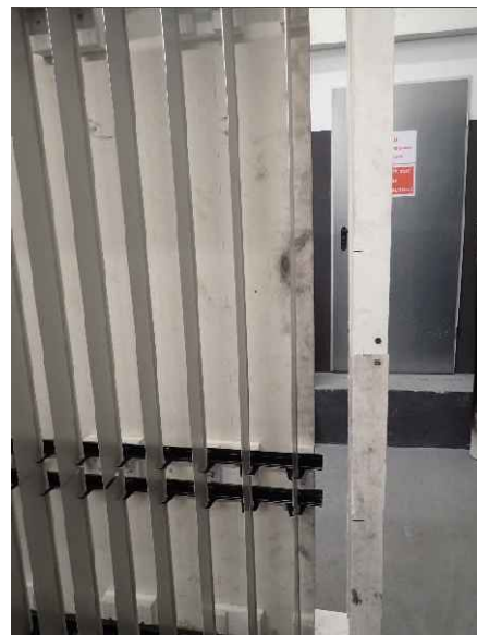
Foto 22: Prüfkörper DZ3.1/23-067V („V-200“), Detailansicht der Außenkante des breiten Probenflügels in Höhe von 500 mm in einem Winkel von ca. 45° vor der Brandprüfung.
